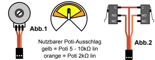
Verdrahtung Poti (Schleifer = rot) Verdrahtung Endlagenschalter (Schließer = NO = normally open)
