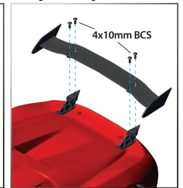
Montage des Kotflügels für 160 km/h (100 mph)
